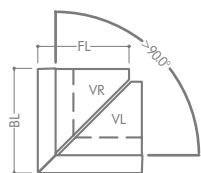
Variable Außenecke, 2 teilig Standard-BL = 40* – 88 cm – Sicht außen, Sicht innen max. BL = 288 – Sicht beidseitig Sonder BL > 88 cm – Sicht außen
