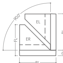
Außenecke, 1 teilig BL = 50 cm, beidseitig Sichtbeton
